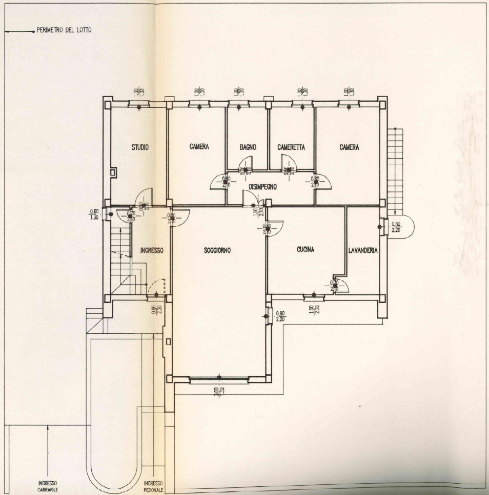
PIANTA PIANO RIALZATO
