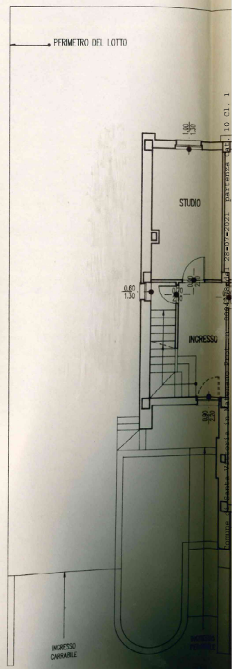
PIANTA PIANO RIALZATO
