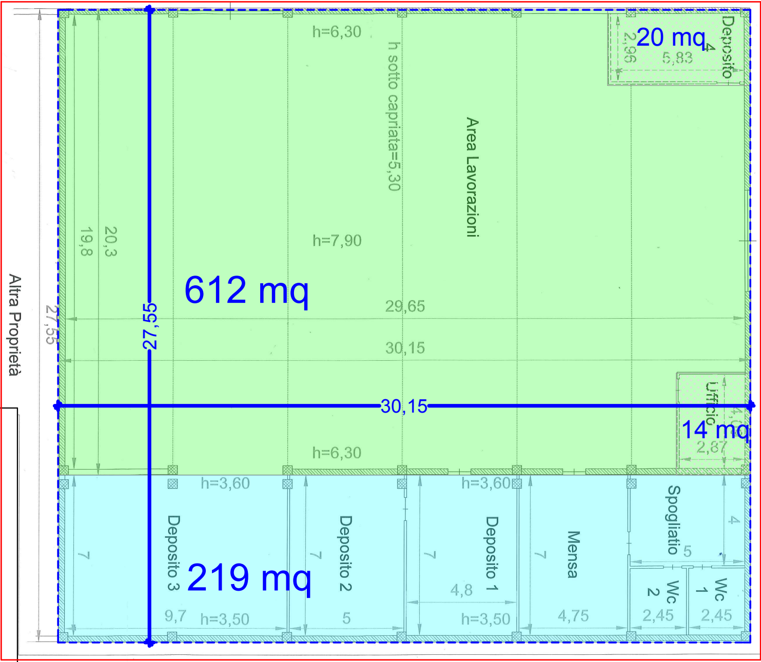
Verifica dati metrici e superfici (su base rilievo geom. Tornillo)
